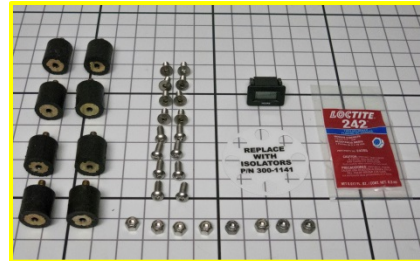
EDGE 32" DC Scrubbers
