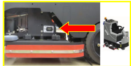
EDGE GTX
